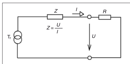
Obr. 4. Princip měření impedance smyčky
