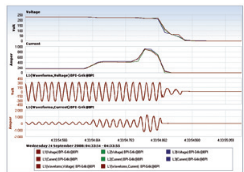
Obr. 5.d Napětí a proud na začátku výpadku (v horní části trend v dolní skutečné časové průběhy)
