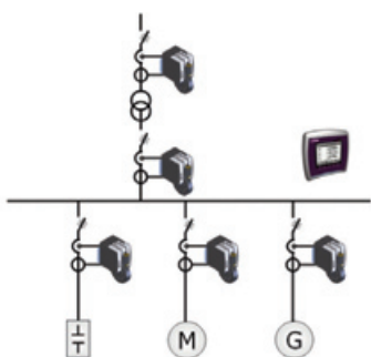
Obr. 1 Umístění ELSPEC G4000 v distribuční síti
