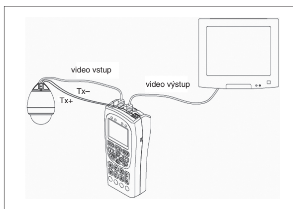
Obr. 3. Zapojení v režimu testu videesignálu
