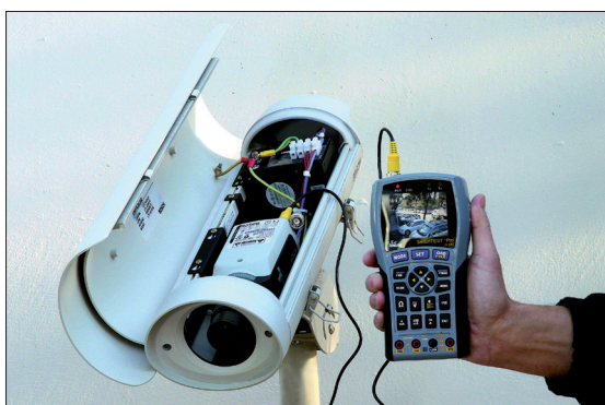
Obr. 1. Použití přístroje SecuriTEST Pro
