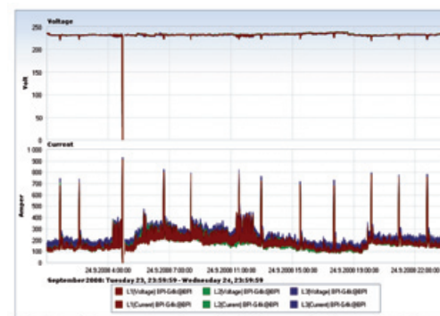
Obr. 5.b Denní záznam (trend napětí a proudu), 24.9.08 po čtvrté hodině ráno dochází k výpadku
