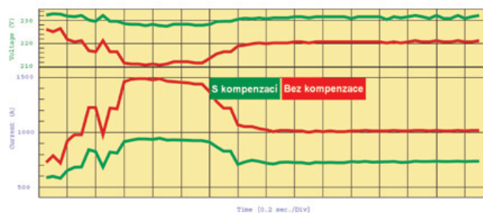
Obr. 7 Porovnání průběhu napětí a zátěžného proudu bez kompenzace a s kompenzací pomocí Equalizeru ELSPEC
