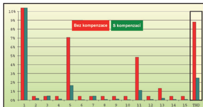
Obr. 8 Filtrační účinek harmonických složek napětí Equalizeru ELSPEC
