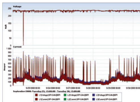
Obr. 5.a Týdenní záznam (trend napětí a proudu)
