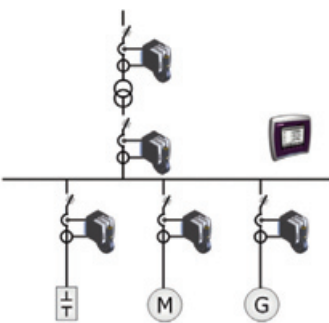
Obr. 1 Umístění ELSPEC G4000 v distribuční síti
