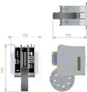
Obr. 2 Analyzátor ELSPEC G4000
