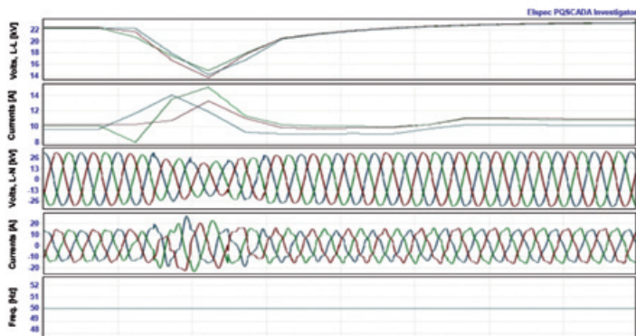
Obr. 4 Záznam poklesu napětí o délce tří period
