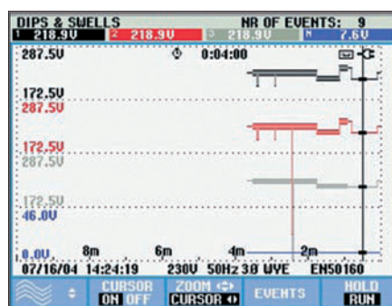
Obr. 9. Průběh křivek indikujících zdroje flickeru
