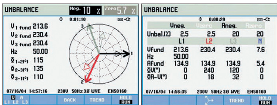
Obr. 10. Zobrazení nevyváženosti sítě
