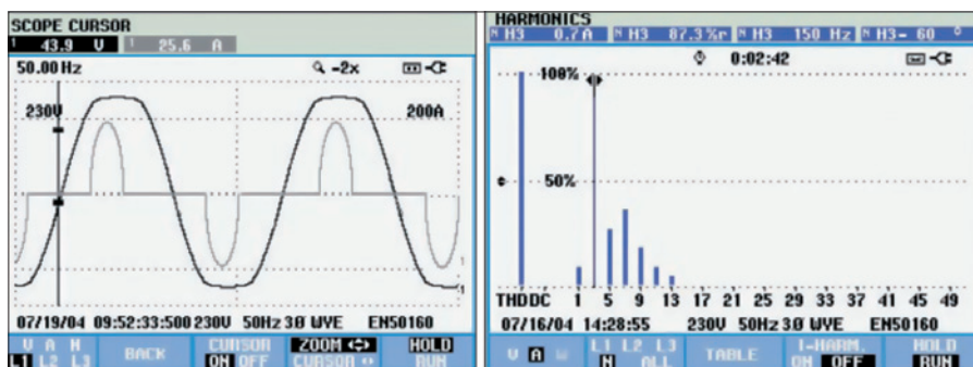
Obr. 4. Typický průběh proudu na usměrňovači a jeho spektrum
